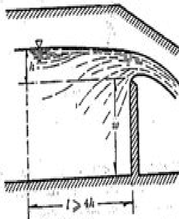
b) Elevación
